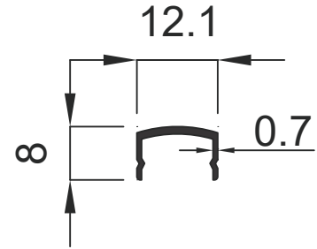
1177 0.060 Kg / m
