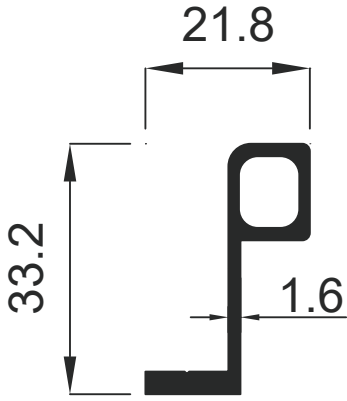
1318 0.352 Kg / m
