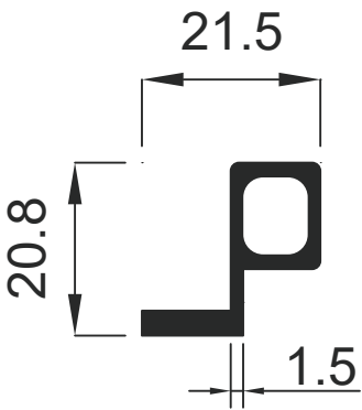
1317 0.301 Kg / m
